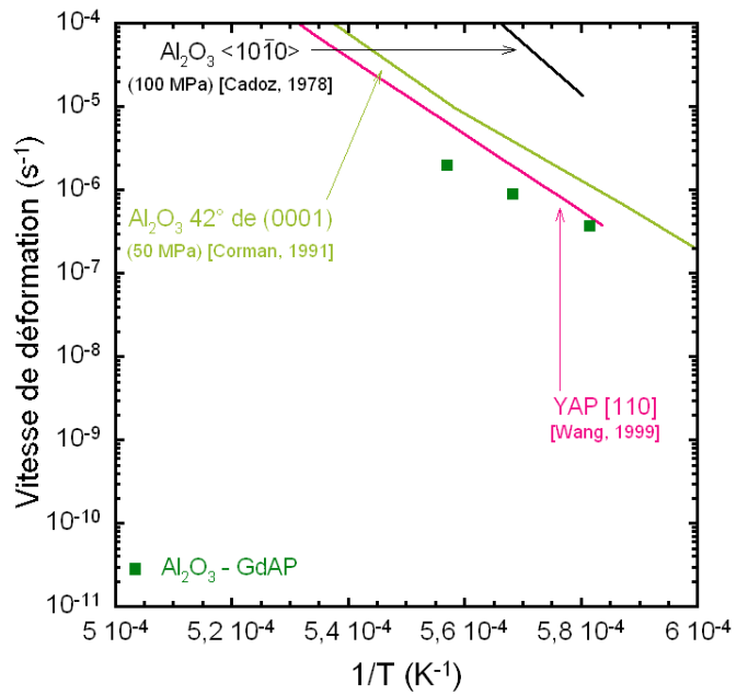
Figure 6.26 Evolution, en fonction de l'inverse de la température, sous une charge de 200 MPa, des vitesses de déformation du YAP et du saphir, comparées à celle du système Al_2O_3 - GdAP.
