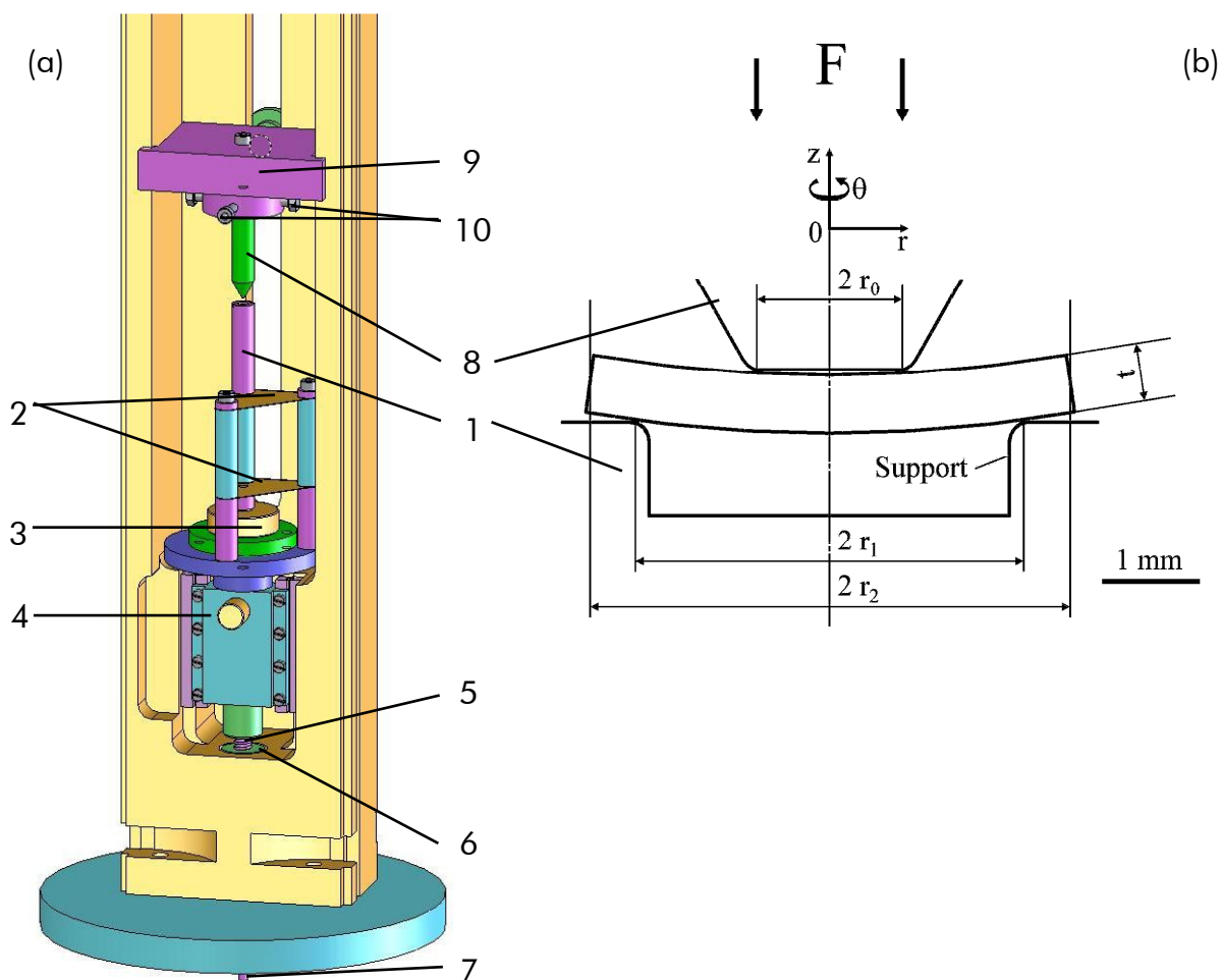
Figure 2.4 (a) Appareil de flexion biaxiale 1 – (b) Epreuve chargée, prise entre le poinçon et le support.
