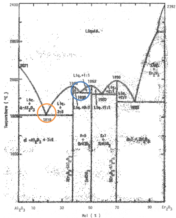
Figure 3.2 Diagramme d'équilibre binaire \text{Al}_2\text{O}_3 - \text{Er}_2\text{O}_3 [Mizuno, 1979].
