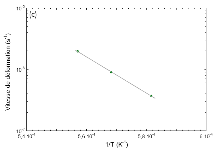
Figure 5.12 Evolution de la vitesse de déformation en fonction de l'inverse de la température pour les eutectiques binaires déformés à 200 MPa : (a) \text{Al}_2\text{O}_3 - YAG, (b) \text{Al}_2\text{O}_3 - ErAG, (c) \text{Al}_2\text{O}_3 - GdAP.
