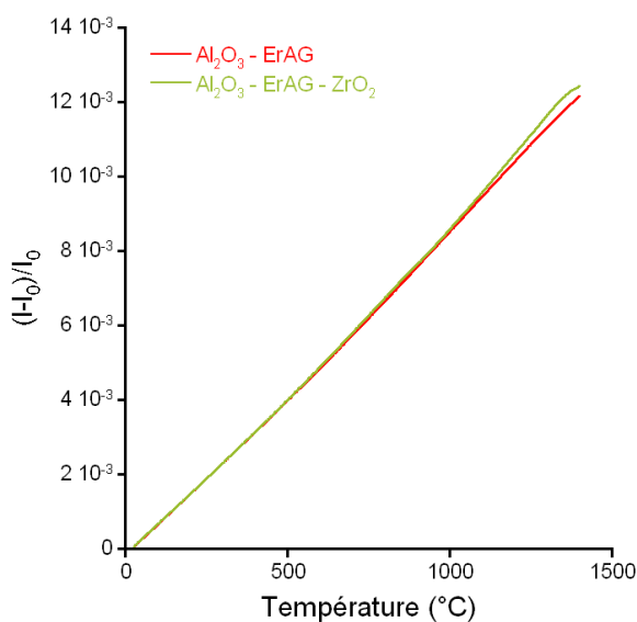
Figure 4.17 Dilatation thermique des composites eutectiques à base d'Er (selon l'axe de croissance).
