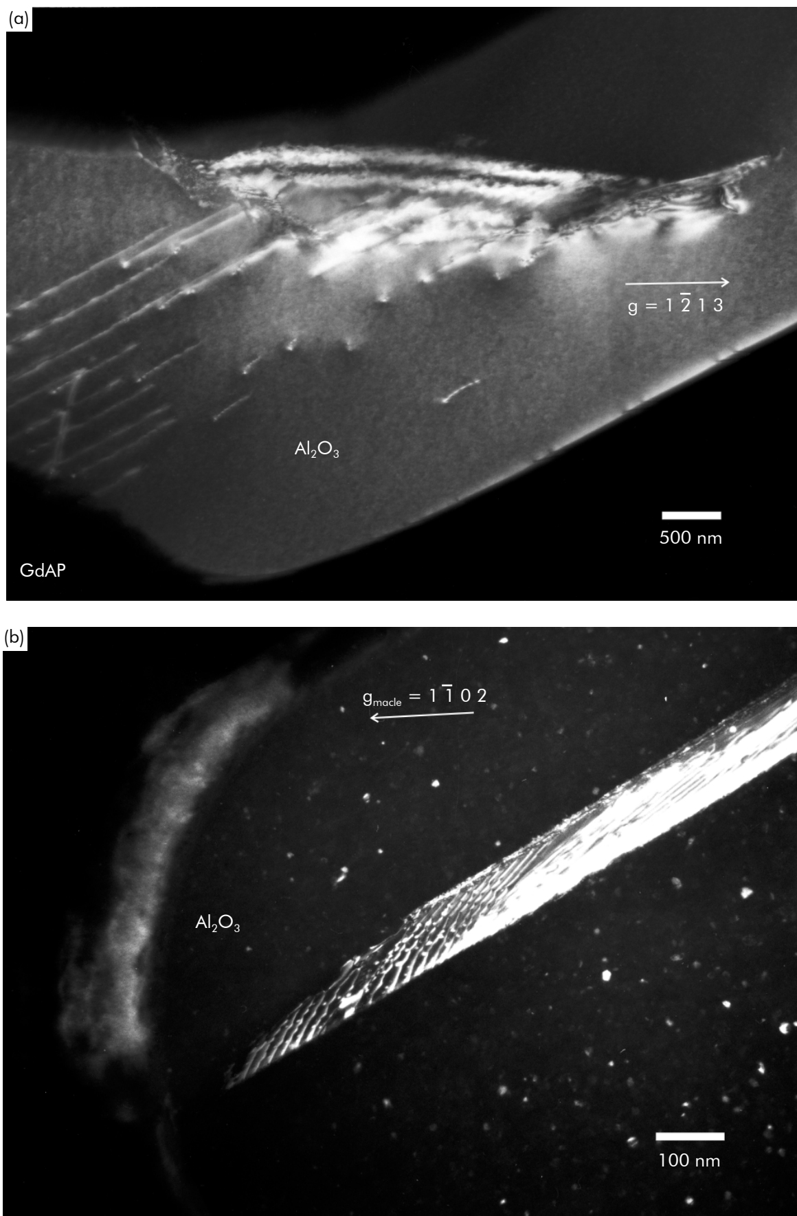
Figure 6.23 Micrographies en champ sombre du composite \text{Al}_2\text{O}_3 - GdAP déformé à 1600^\circ\text{C} : présence de glissement basal (a) et de maclage basal (b) dans la phase \text{Al}_2\text{O}_3 .
