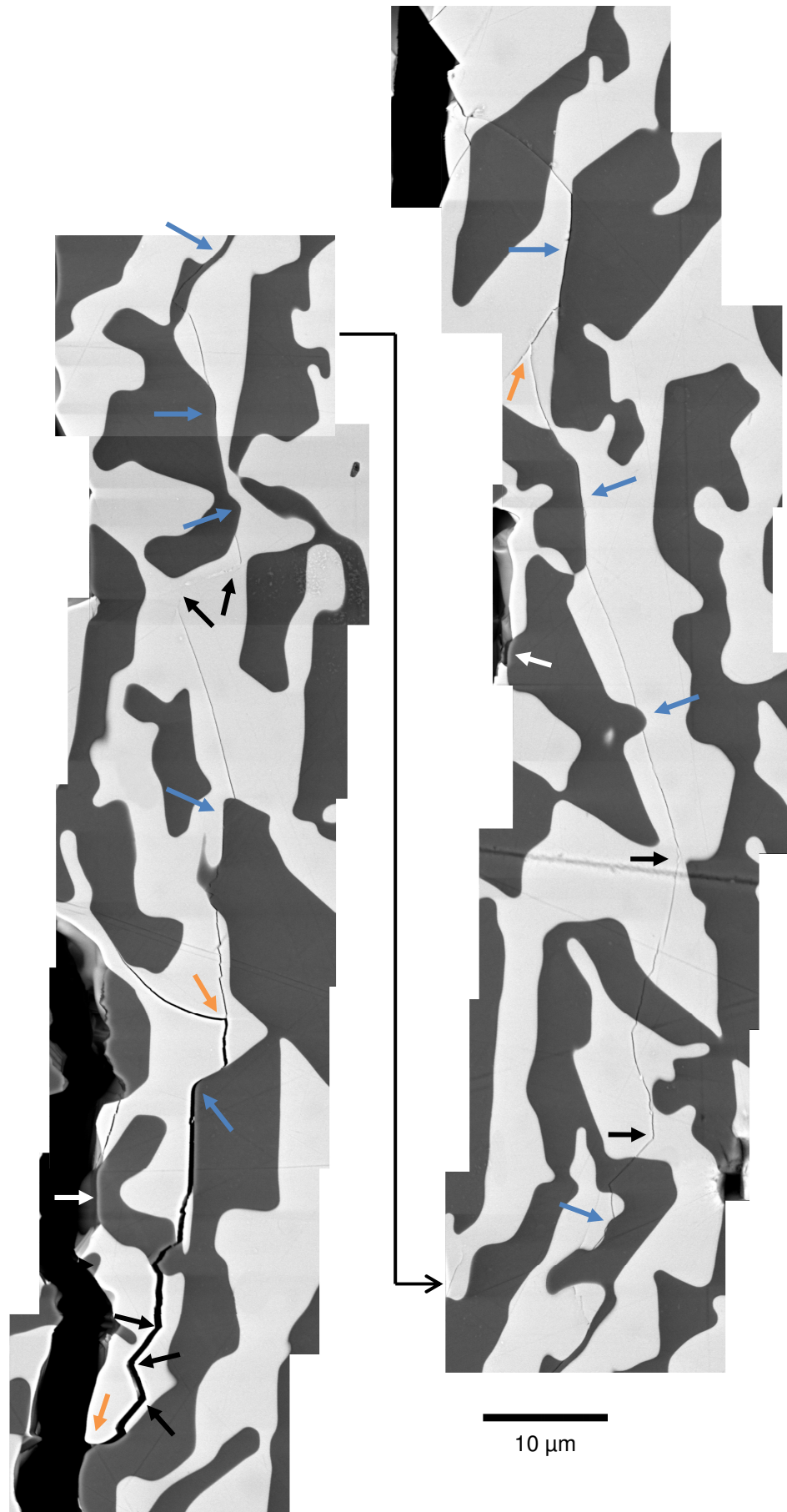
Figure 4.7 Système Al 2 O 3 - YAG : propagation de fissure au sein de la microstructure.
