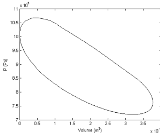
FIG. 1.3 : Diagramme indicateur d'un moteur STIRLING réel
