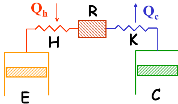
FIG. 5.7 : Configuration typique d'un moteur STIRLING
