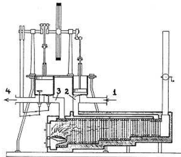
FIG. 5.1 : Moteur thermique de Joule (1851/1852)
