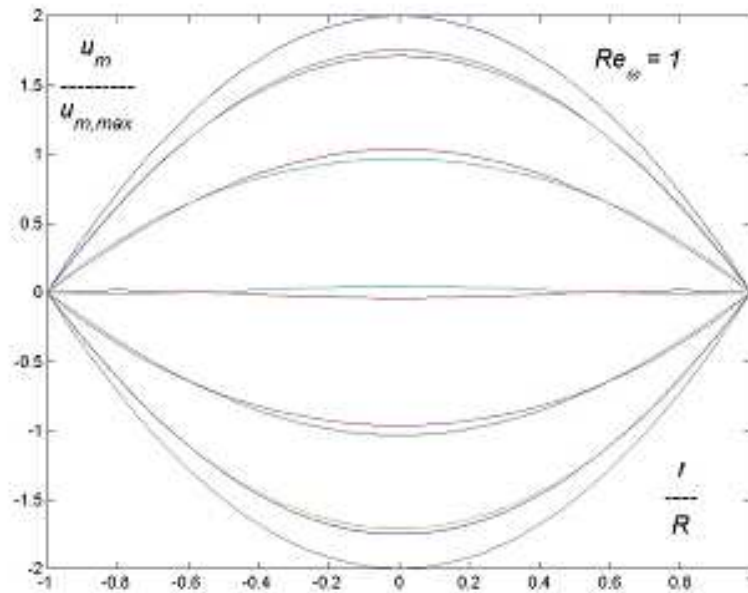
FIG. 3.2 : Profil des vitesses en écoulement laminaire incompressible établi à faible fréquence
