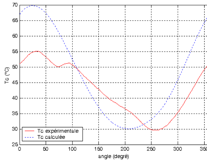
FIG. 3.7 : Evolutions des températures expérimentale et calculée au niveau du cylindre de compression
